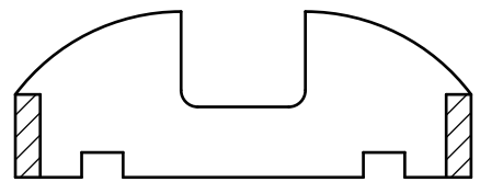
B-B断面(3ヶ所) 基本寸法は正面図と同様
