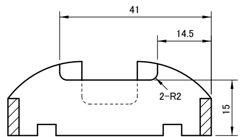
A-A断面(3ヶ所) 基本寸法は正面図と同様
