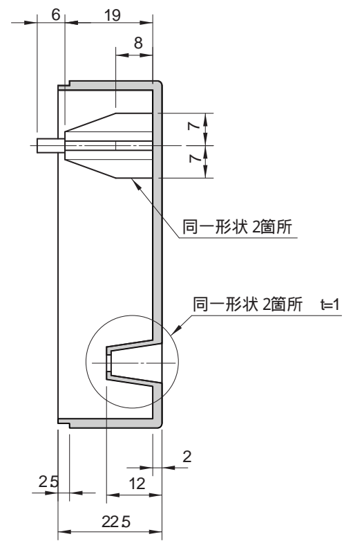
A-A断面
