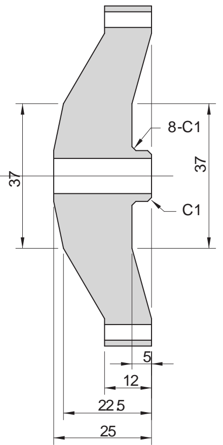
A-A断面
